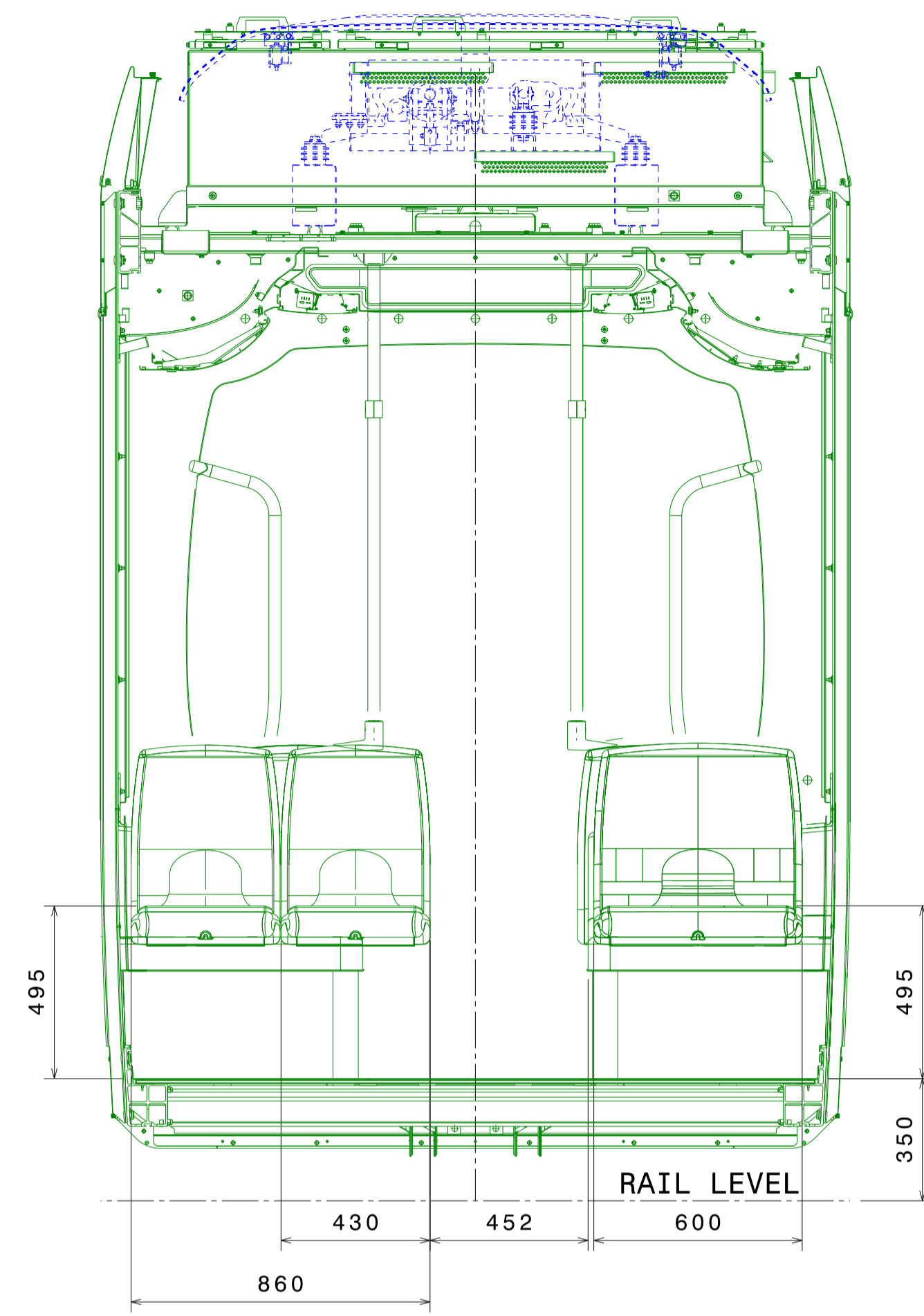
D-D 1:15
