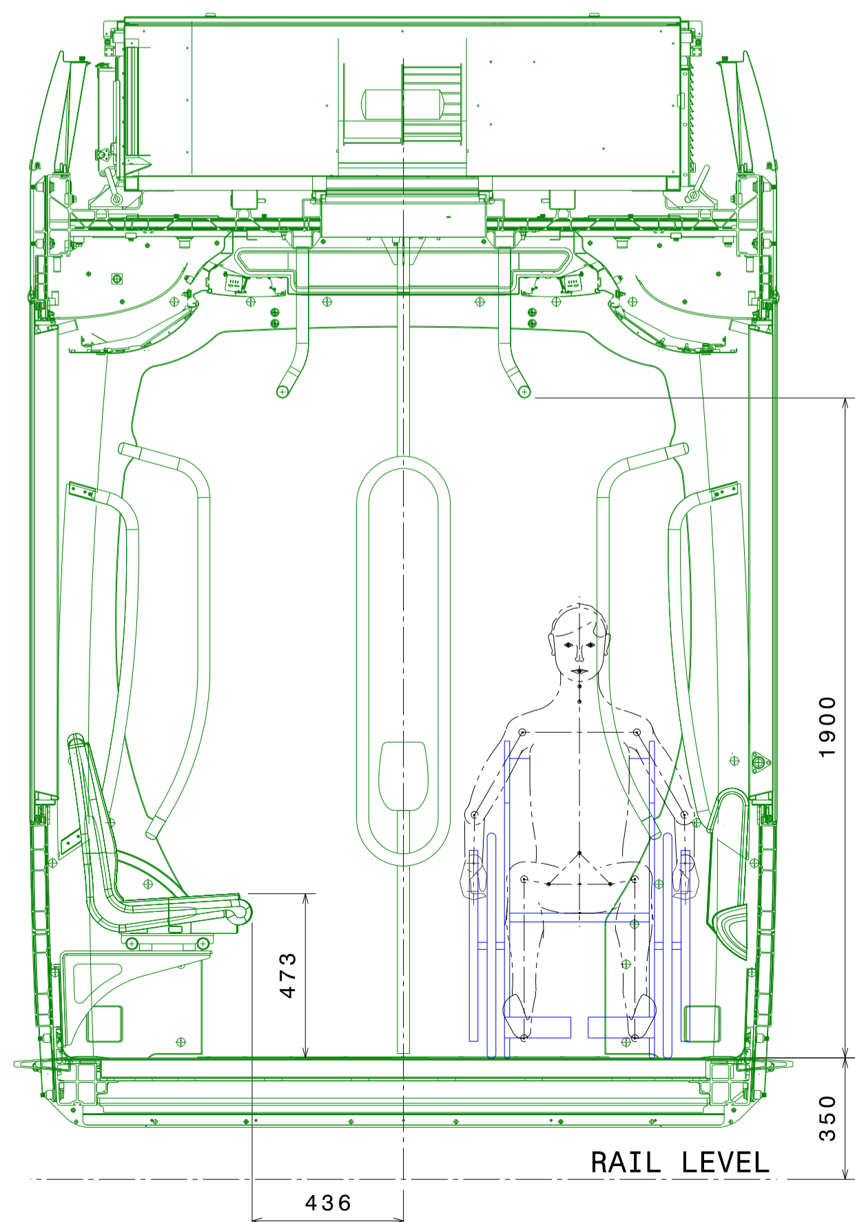
E-E 1:15
