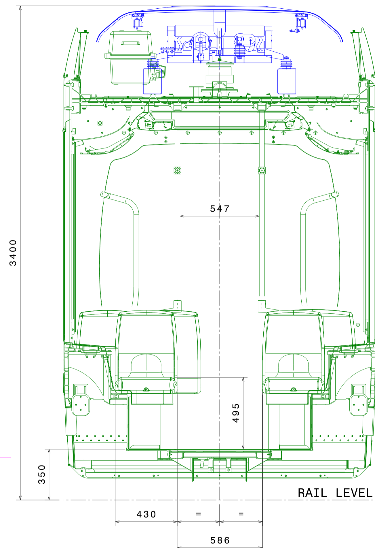
C-C 1:15
